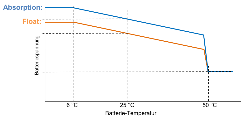
Abbildung 16 Grafik zum Temperatursgleich für die Spannungswerte der Ladeerhaltungs- und Konstant Spannungs-Phasen
