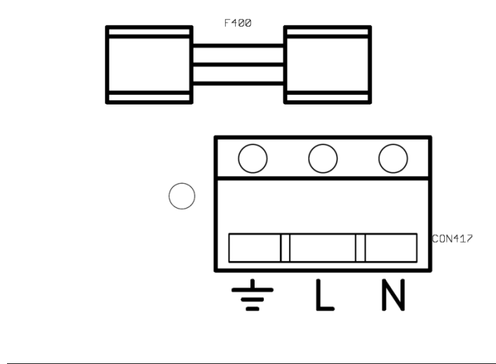
Figura 22 Morsetto di entrata rete alimentazione
