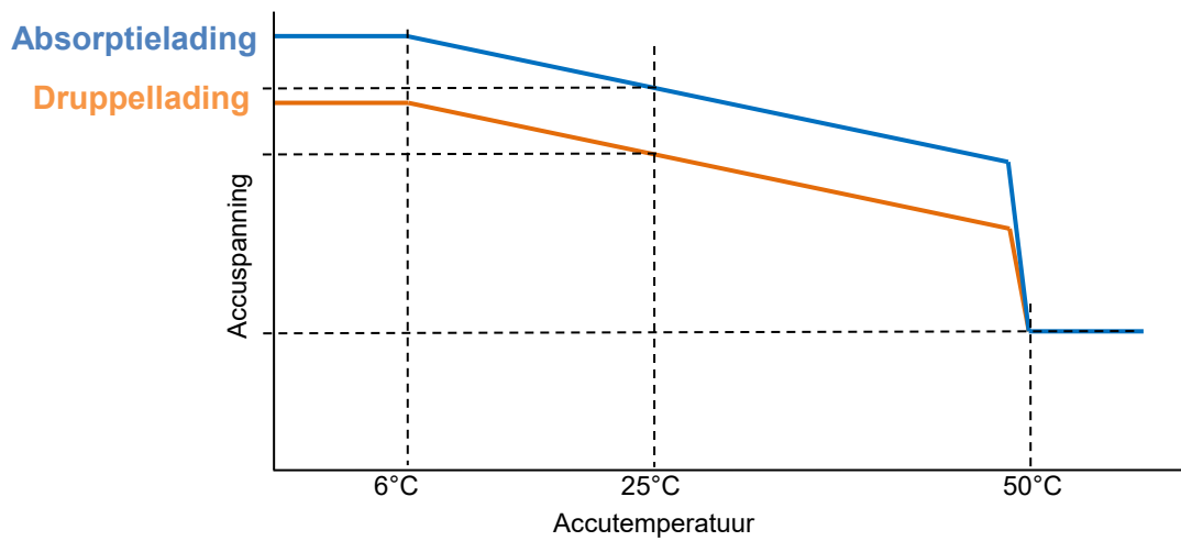
Afbeelding 8 Temperatuurcompensatiediagram voor druppellading- en absorptiespanningen
