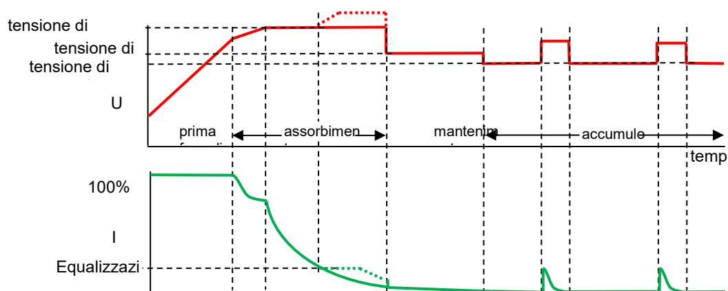
Figura 23 Tensione e corrente durante i vari stadi di carica della batteria
