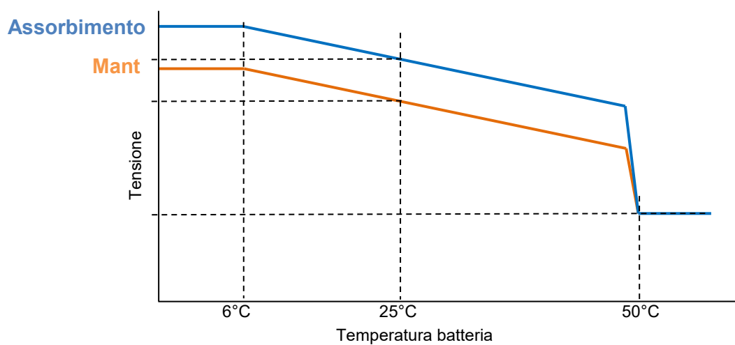
Figura 24 Grafico della compensazione della temperatura per la tensione di assorbimento e di mantenimento
